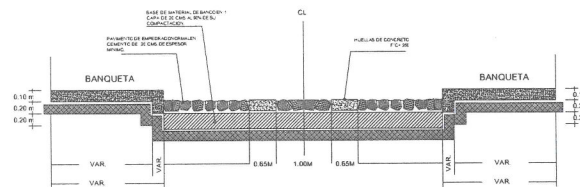
DETALLE CONSTRUCTIVO
