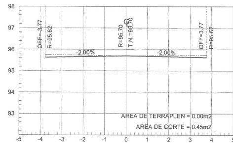
ESTACION 0+000.00 ESCALA HORIZONTAL 1 : 100 ESCALA VERTICAL 1 : 100
