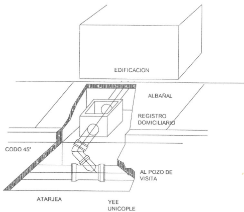
DETALLE DE CONEXIÓN DE ALBAÑAL
