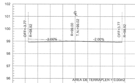
ESTACION 0+060.00 ESCALA HORIZONTAL 1 : 100 ESCALA VERTICAL 1 : 100
