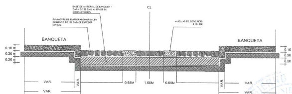
DETALLE CONSTRUCTIVO
