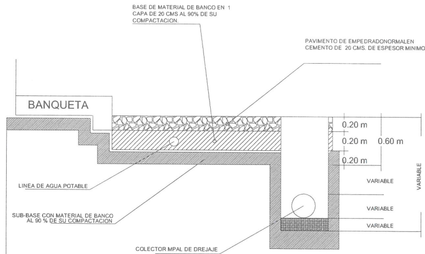
DETALLE CONSTRUCTIVO
