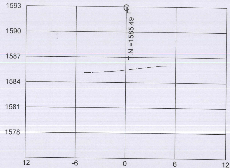
ESTACION 0+056.07 ESCALA HORIZONTAL 1 : 100 ESCALA VERTICAL 1 : 100
