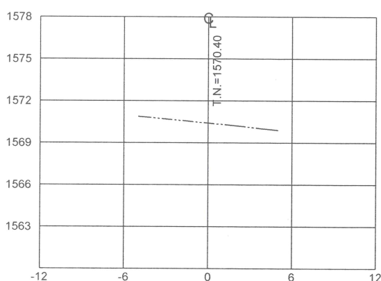
ESTACION 0+060.00 ESCALA HORIZONTAL 1 : 100 ESCALA VERTICAL 1 : 100
