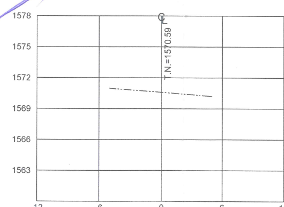
ESTACION 0+165.00 ESCALA HORIZONTAL 1 : 100 ESCALA VERTICAL 1 : 100
