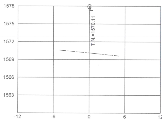
ESTACION 0+080.00 ESCALA HORIZONTAL 1 : 100 ESCALA VERTICAL 1 : 100
