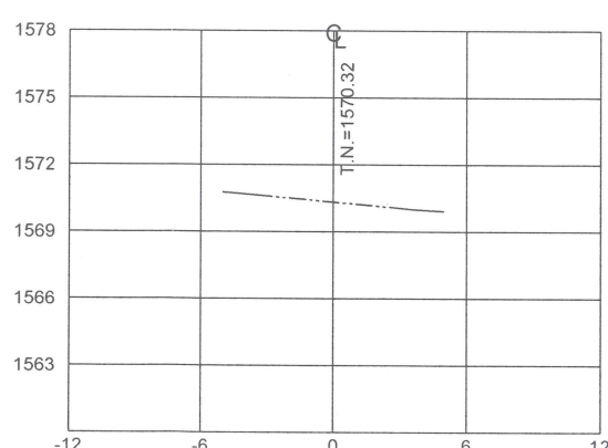
ESTACION 0+120.00 ESCALA HORIZONTAL 1 : 100 ESCALA VERTICAL 1 : 100
