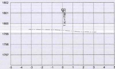
ESTACION 0+060.00 ESCALA HORIZONTAL 1 : 100 ESCALA VERTICAL 1 : 100
