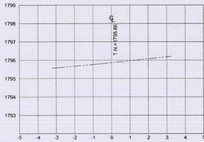
ESTACION 0+040.00 ESCALA HORIZONTAL 1 : 100 ESCALA VERTICAL 1 : 100
