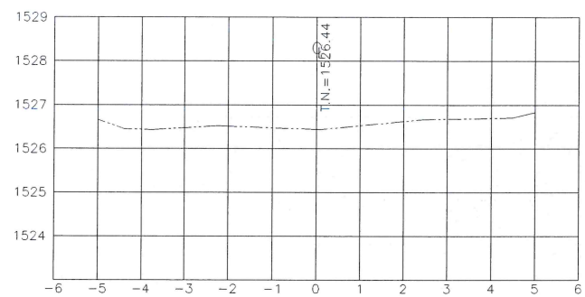
ESTACION 0+010.00 ESCALA HORIZONTAL 1 : 100 ESCALA VERTICAL 1 : 100
