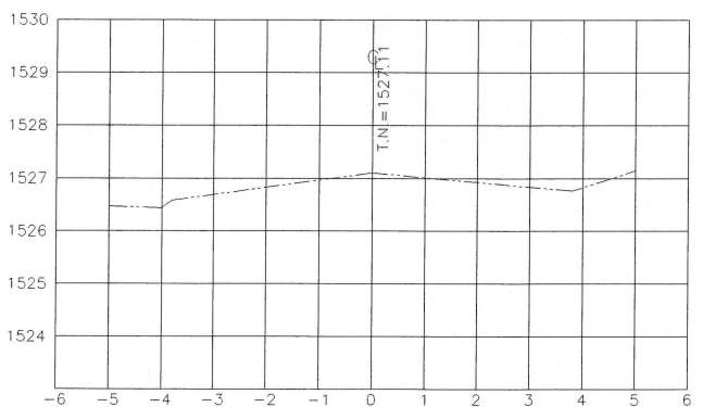
ESTACION 0+000.00 ESCALA HORIZONTAL 1 : 100 ESCALA VERTICAL 1 : 100
