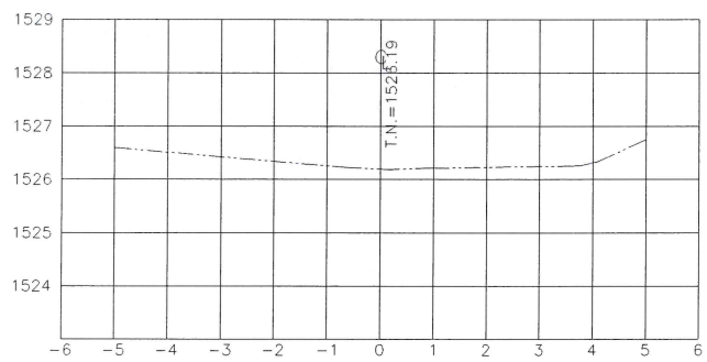
ESTACION 0+025.00 ESCALA HORIZONTAL 1 : 100 ESCALA VERTICAL 1 : 100
