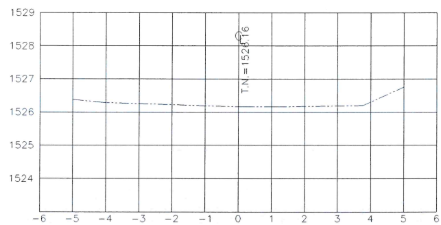
ESTACION 0+028.47 ESCALA HORIZONTAL 1 : 100 ESCALA VERTICAL 1 : 100
