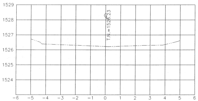
ESTACION 0+020.00 ESCALA HORIZONTAL 1 : 100 ESCALA VERTICAL 1 : 100
