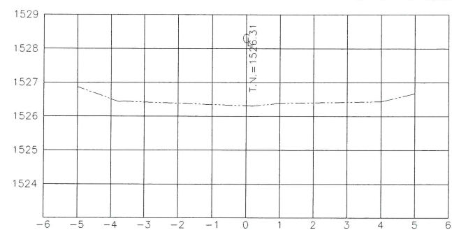
ESTACION 0+015.00 ESCALA HORIZONTAL 1 : 100 ESCALA VERTICAL 1 : 100
