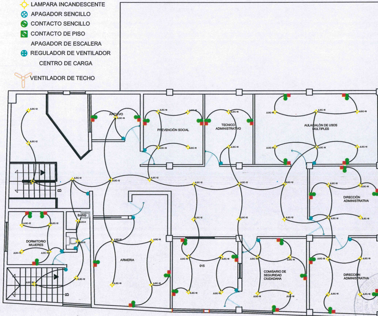
PLANTA ALTA
