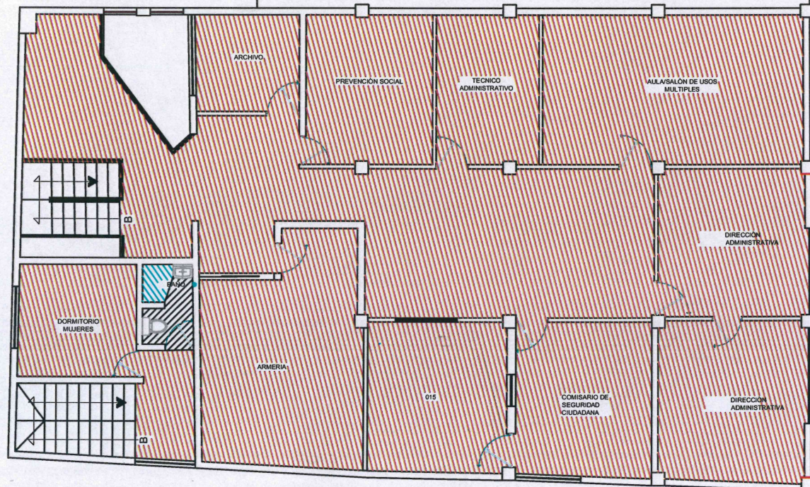
PLANTA ALTA
