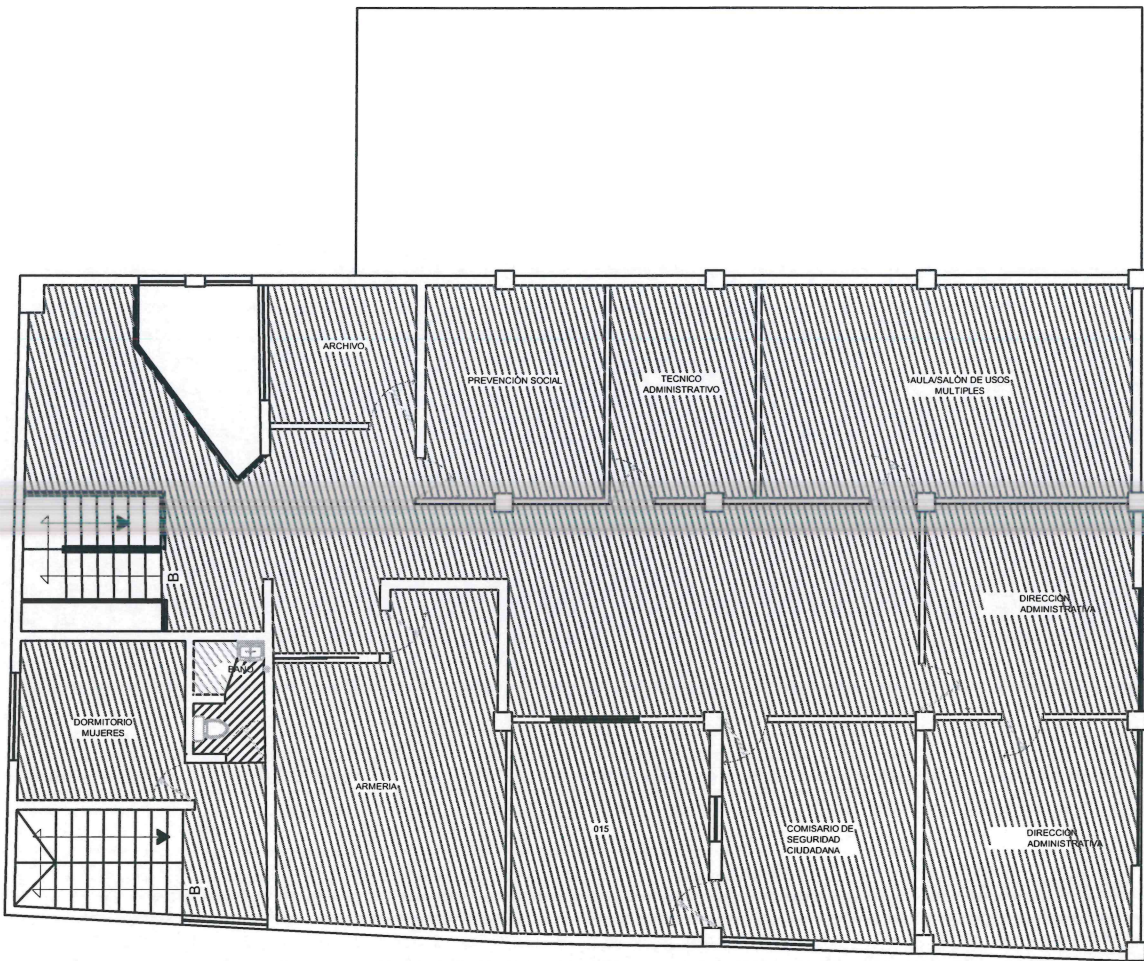
PLANTA ALTA
