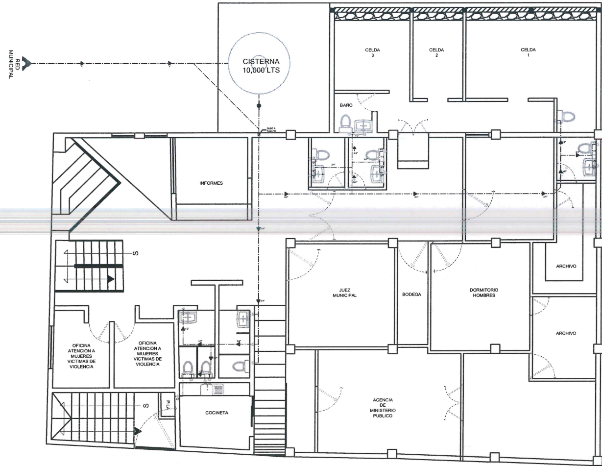
PLANTA BAJA
