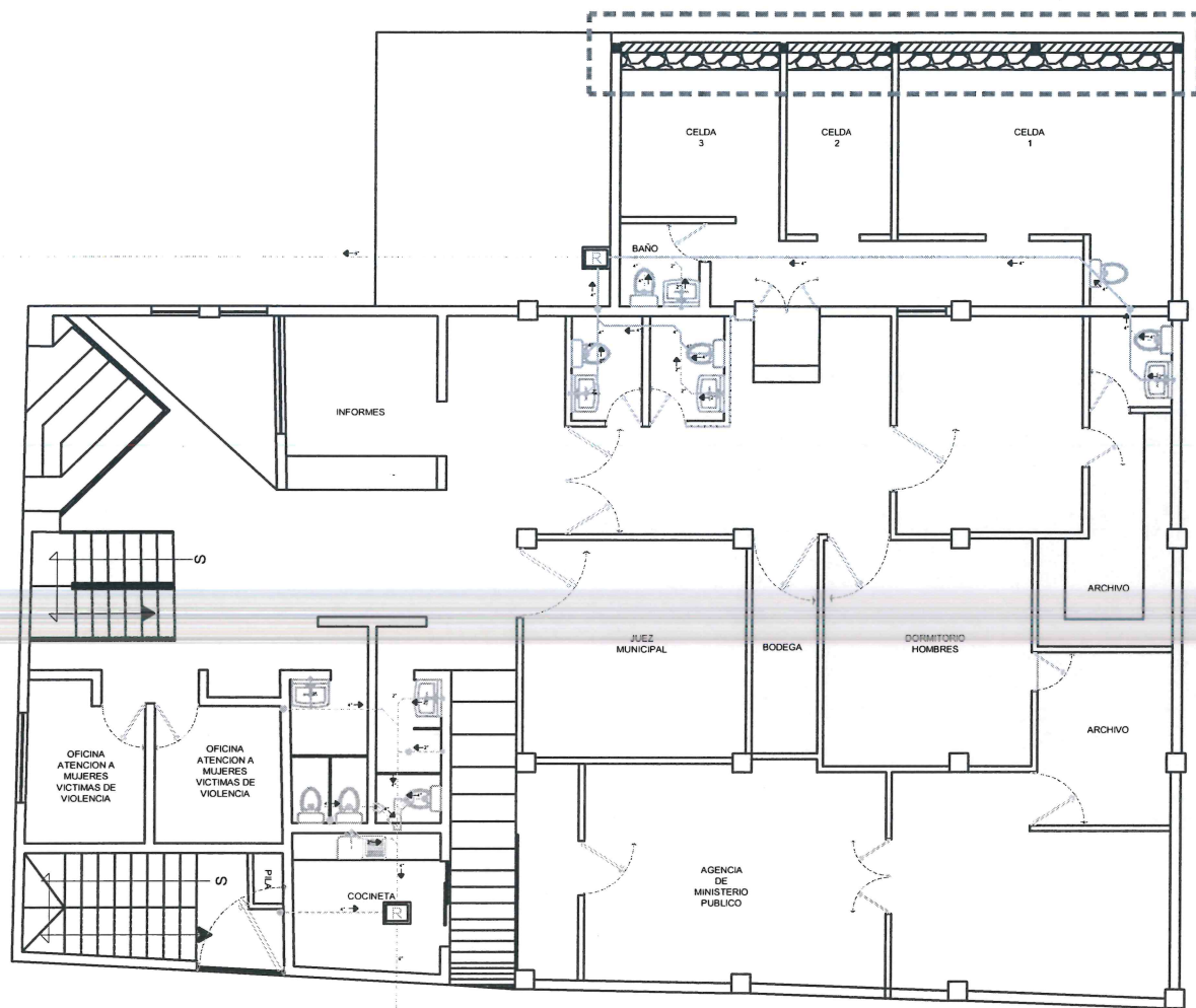
PLANTA BAJA
