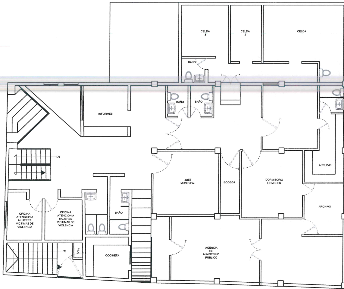
PLANTA BAJA ESTADO ACTUAL
