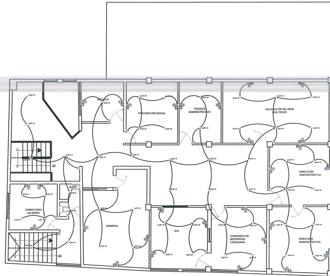
PLANTA ALTA
