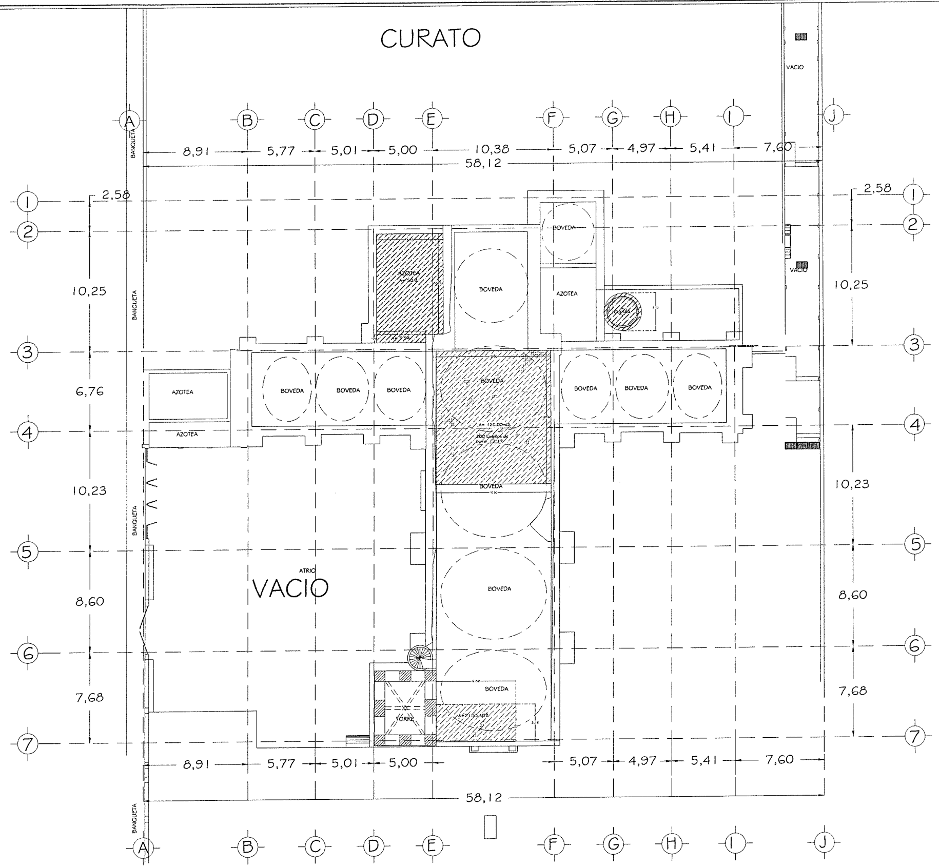
CROQUIS DE TRABAJOS DE IMPERMEABILIZACIÓN EN BOVEDAS DEL TEMPLO DEL SR. DEL MONTE
