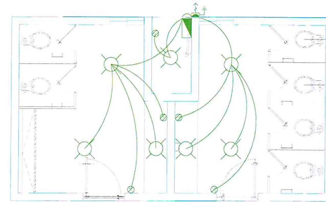
SÍMBOLOGIA INSTALACIÓN ELÉCTRICA
