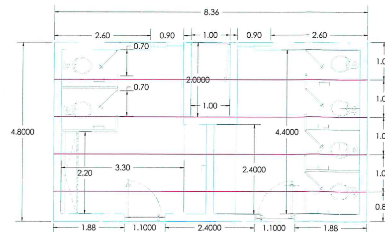
Planta de Viguería
