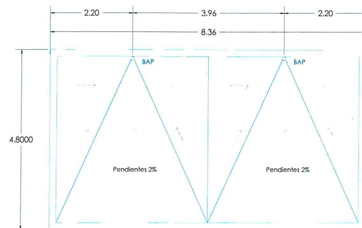
Planta de Azotea
