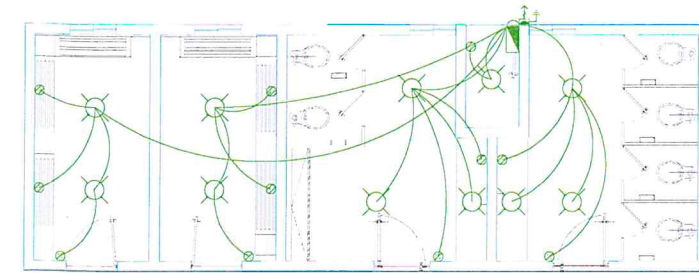
Planta de Instalación Eléctrica
