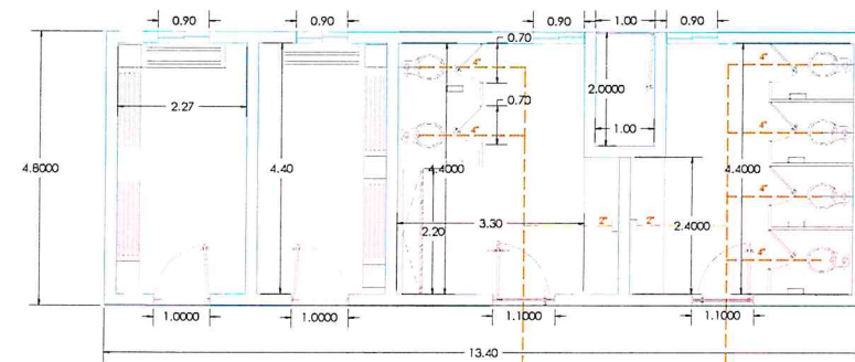
Planta Arquitectónica
