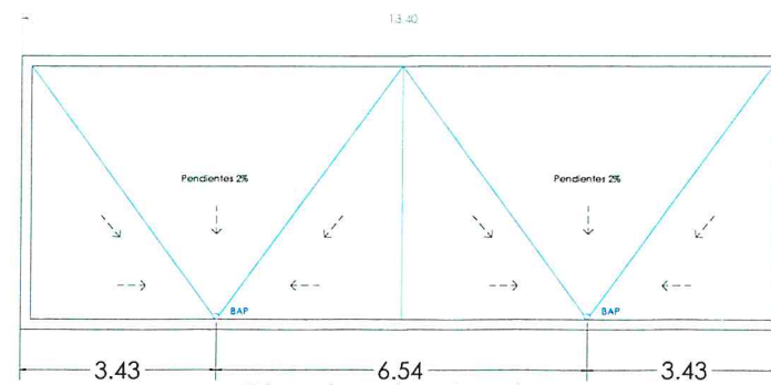
Planta de Azotea
