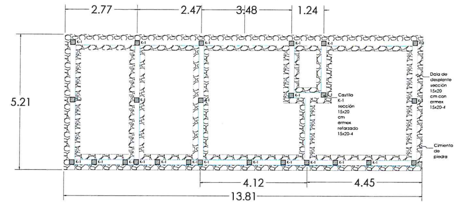
Planta de Cimentación
