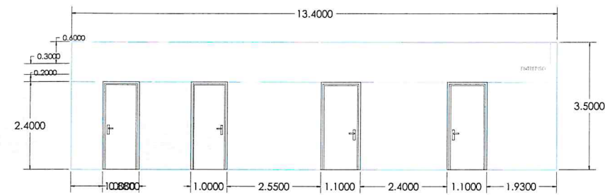
Elevación frontal
