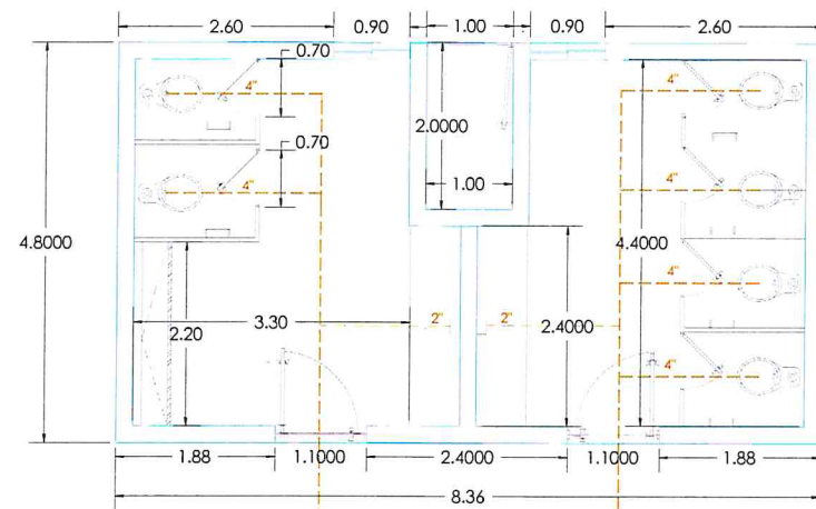
Planta Arquitectónica
