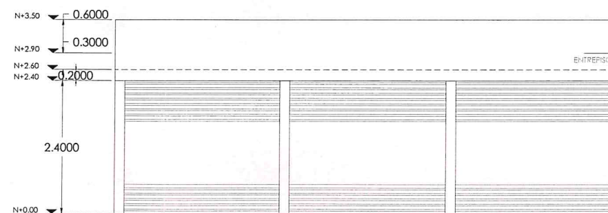
Elevación frontal
