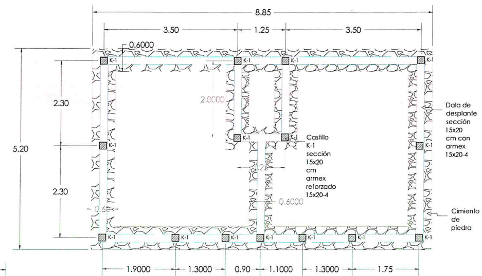
Planta de Cimentación
