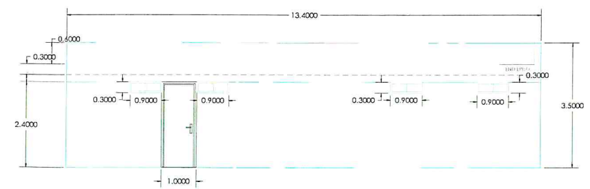
Elevación posterior
