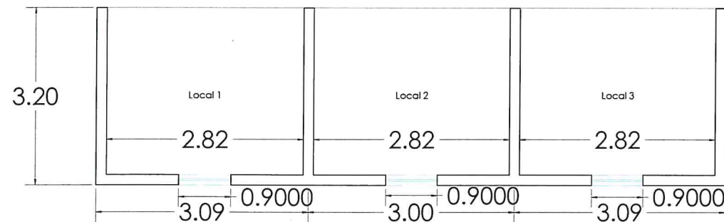
Planta Arquitectónica
