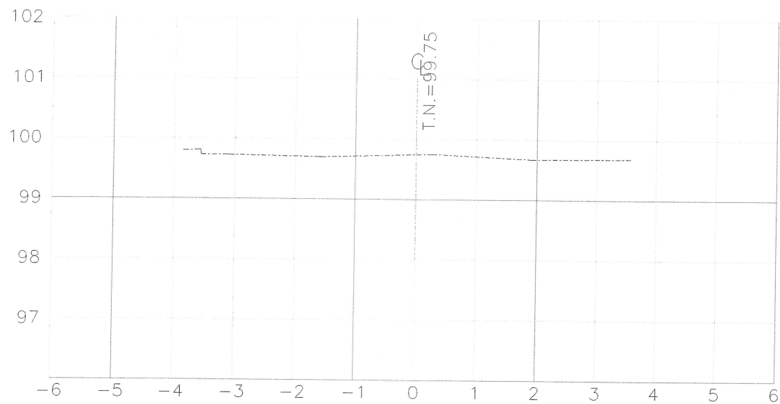
ESTACION 0+010.00 ESCALA HORIZONTAL 1 : 100 ESCALA VERTICAL 1 : 100
