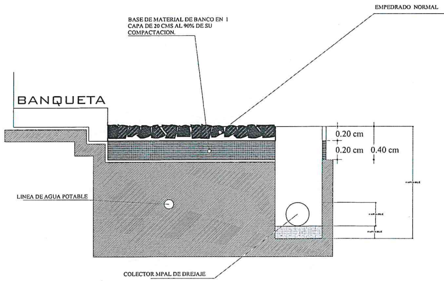
DETALLE CONSTRUCTIVO
