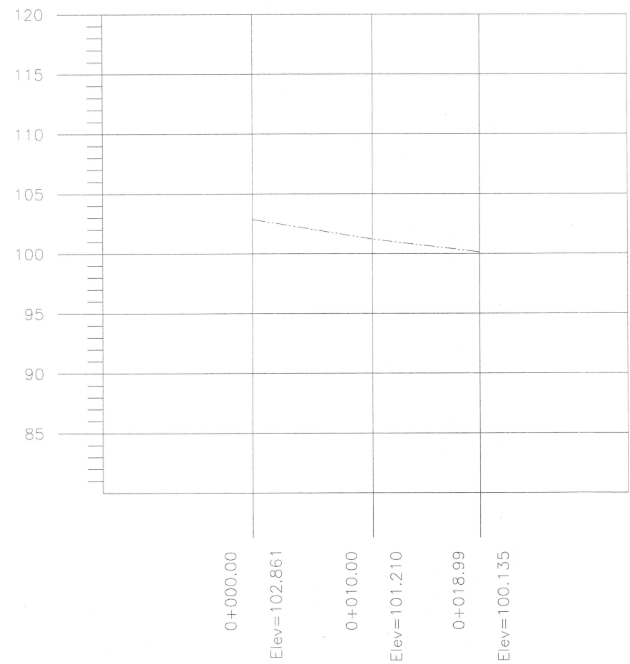
PERFIL 1 ESCALA HORIZONTAL 1 : 1000 ESCALA VERTICAL 1 : 1000
