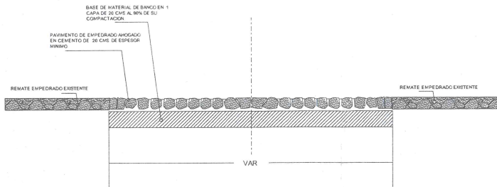
DETALLE CONSTRUCTIVO
