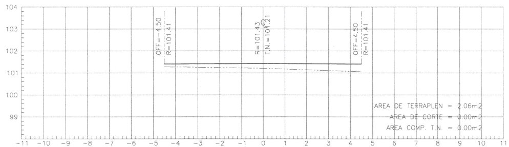
ESTACION 0+010.00 ESCALA HORIZONTAL 1 : 100 ESCALA VERTICAL 1 : 100
