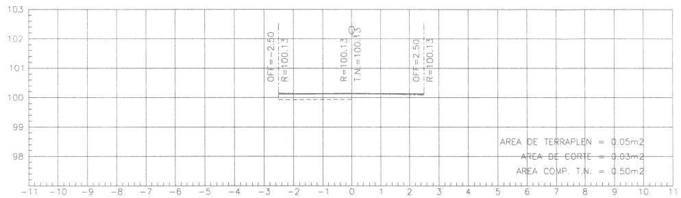
ESTACION 0+019.00 ESCALA HORIZONTAL 1 : 100 ESCALA VERTICAL 1 : 100
