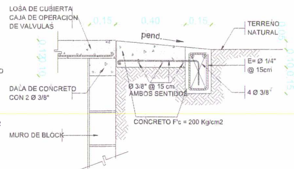
LOSA DE PROTECCIÓN ( PROTECCION PERIMETRAL )
