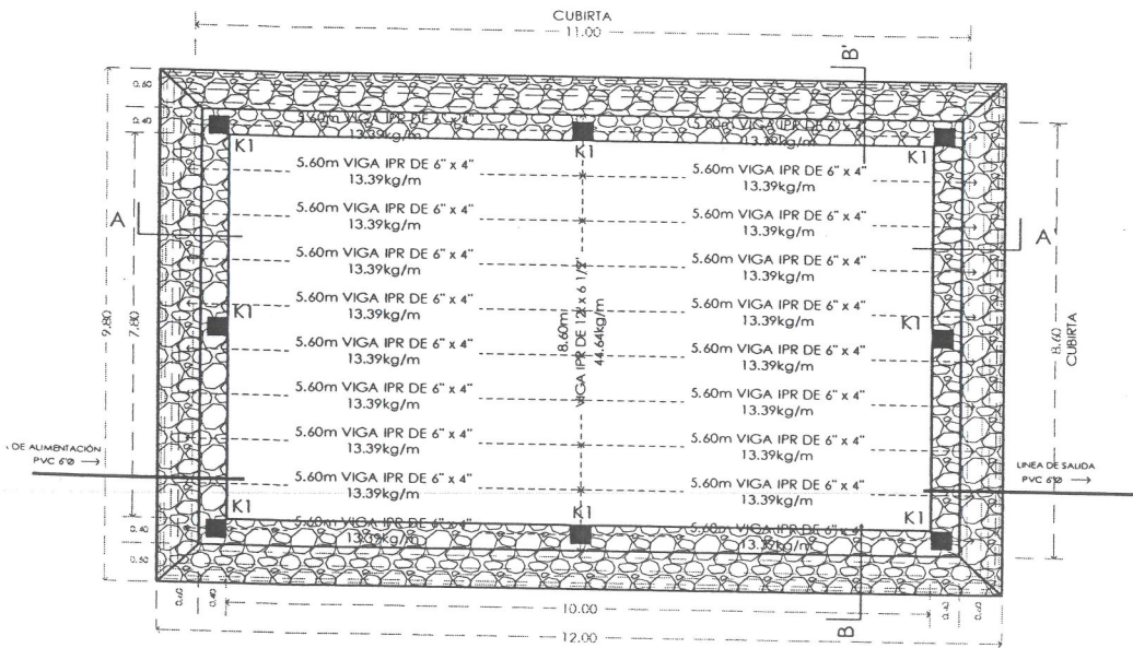
PLANTA DEL DEPOSITO
