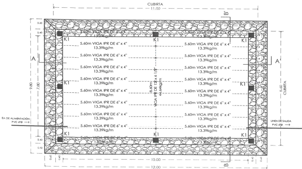
PLANTA DEL DEPOSITO
