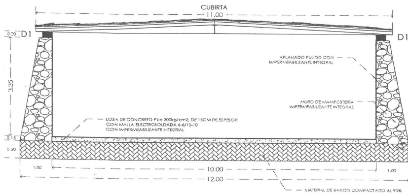
SECCIÓN A, A'
