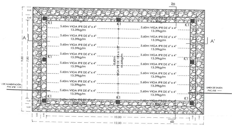
PLANTA DEL DEPOSITO
